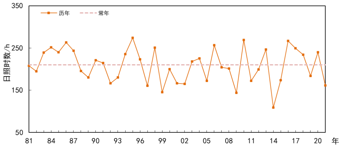
宁波市8月日照时数年际变化图
