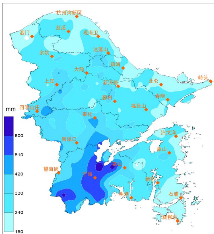
宁波市 2021 年 8 月降水量空间分布图
