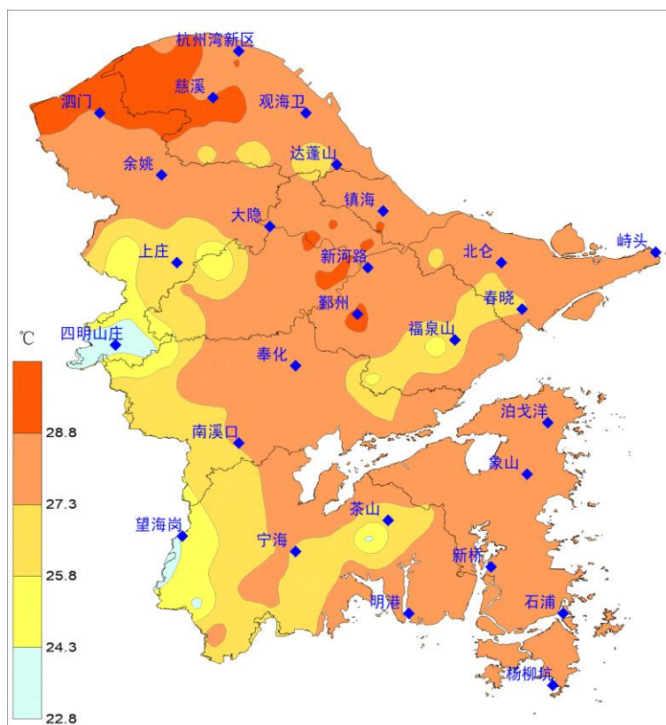
宁波市 2021 年 8 月平均气温空间分布图
