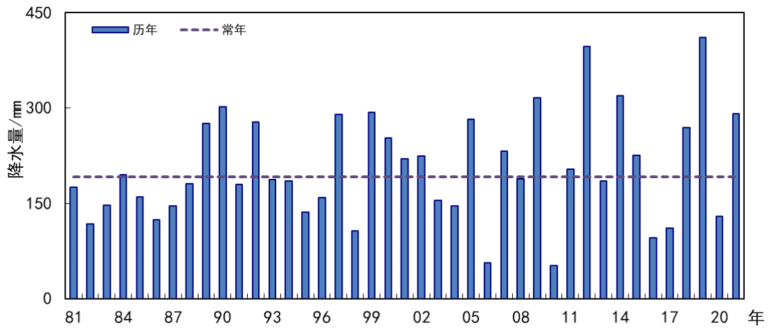
宁波市8月降水量年际变化图
