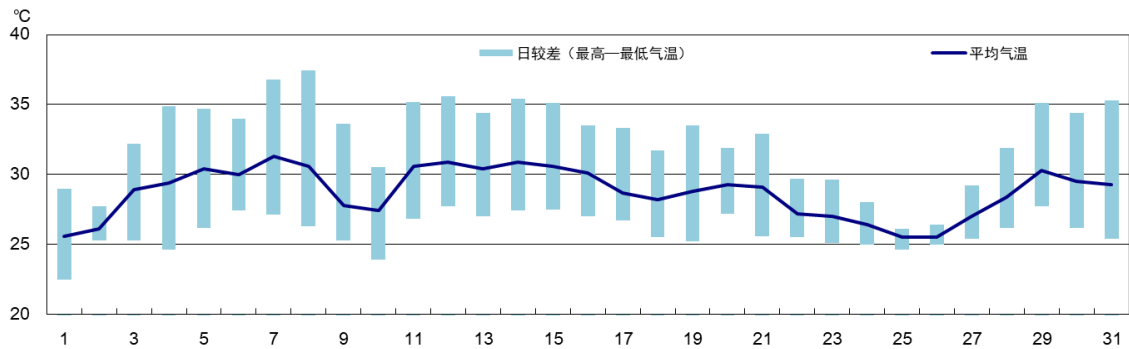
2021 年 7 月鄞州国家基本气象站日平均气温和气温日较差变化图
