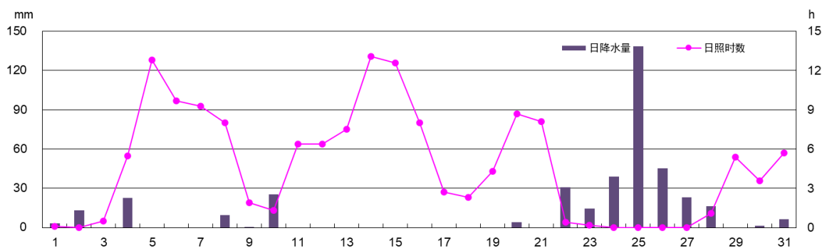
2021年7月鄞州国家基本气象站日降水量和日照时数变化图
